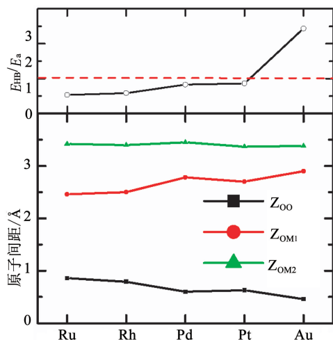
图6 金属表面上水双层(H向上)的结构参数和浸润能力( E_{HB}/E_a )比较(其中 Z_{OO} 是水双层的厚度(即两个氧原子之间的垂直距离), Z_{OM} 是氧原子和金属原子之间的垂直距离, E_a 为吸附能, E_{HB} 为氢键能)
