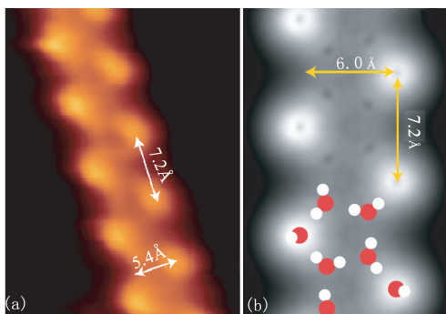
图 4 Cu(110) 表面上由水五元环组成的链状结构图像 (a) 实验 STM 图像; (b) 理论模拟图像及分子结构(引自文献 [27] )
