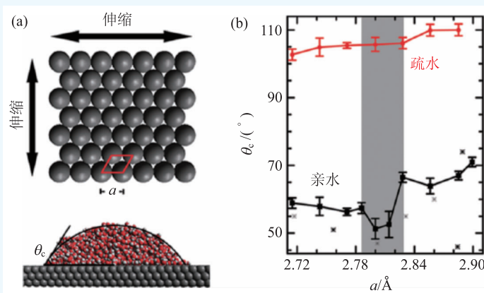
图3 (a)计算模型：通过计算不同晶格常数上的接触角来研究晶格变化对浸润的影响，接触角是由通过拟合水滴在衬底上的侧视图得到；(b)接触角随晶格常数的变化
