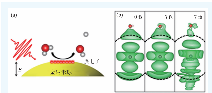
图6 (a)在脉冲激光作用下，金纳米颗粒等离激元诱导的水分解示意图，图中双箭头标记电场 E 的极化方向；(b)费米能级处体系电荷密度的含时演化，图中虚线代表纳米颗粒的表面，灰点代表纳米颗粒中心
