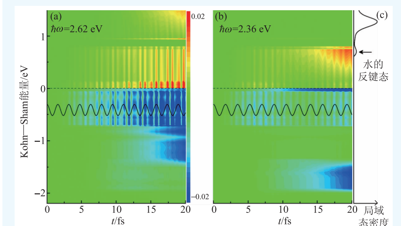
图7 在激光频率2.62 eV(a)和2.36 eV(b)作用下电子占据数的含时演化，图中水平虚线代表费米能级，黑线代表外场演化；(c)整个体系水分子的局域态密度
