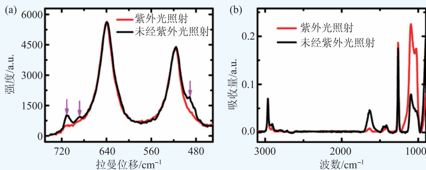
图2 TiO 2 /PMDS的拉曼光谱(a)和红外光谱(b)表征
