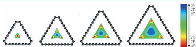
图5 水分子在石墨炔三角形纳米孔中的势能分布(从左到右: n=3, 4, 5, 6 )
